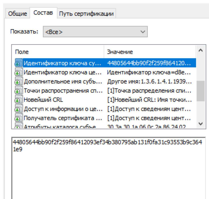
Вибір поля «Идентификатор ключа субъекта» (рис. 6)
